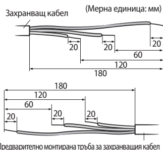
Предварително монтирана тръба за захранващ кабел
